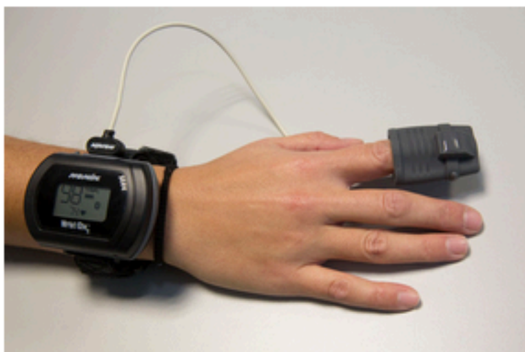
Pulsoxímetro portátil para medir la frecuencia cardíaca y la saturación de oxígeno durante el sueño/ UCC+I Universitat Jaume I
